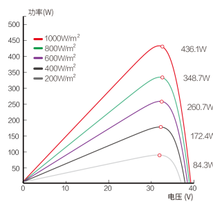
功率-电压曲线 (435W) Cells temp.=25°C
