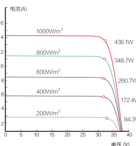
电流-电压曲线 (435W) Cells temp.=25°C
